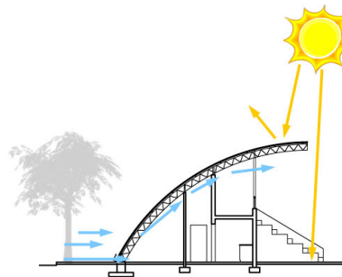
VERANO - ENFRIAMIENTO PASIVO SUMMER - PASSIVE COOLING
