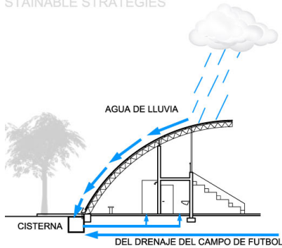
ALMACENAMIENTO DE AGUAS PLUVIALES RAINWATER COLLECTION AND STORAGE
